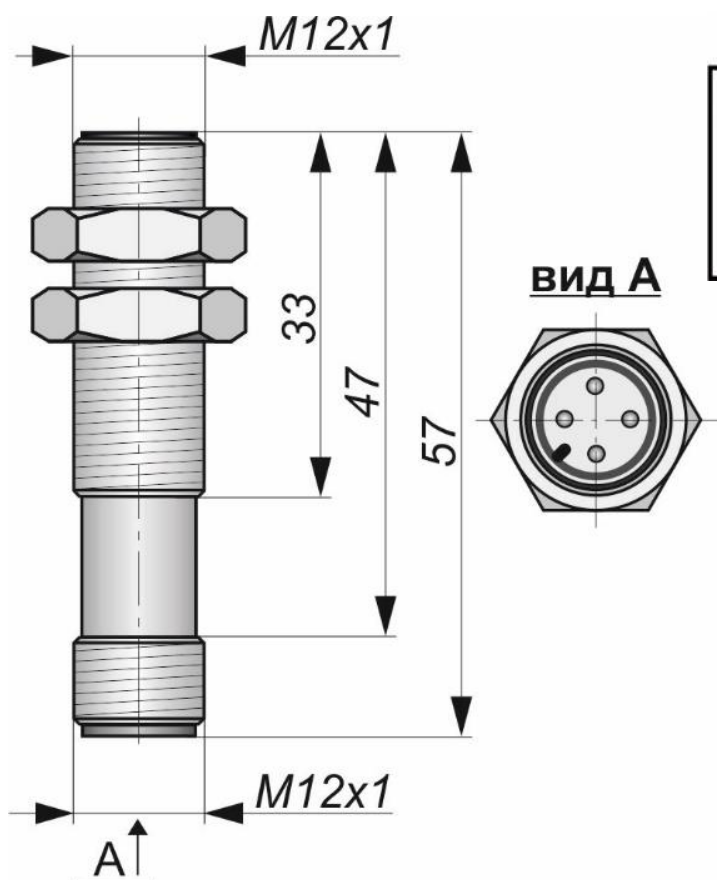
Габаритный чертеж
