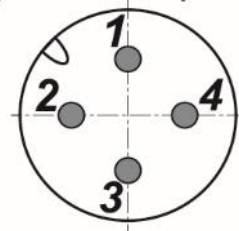
Цоколевка разъема
